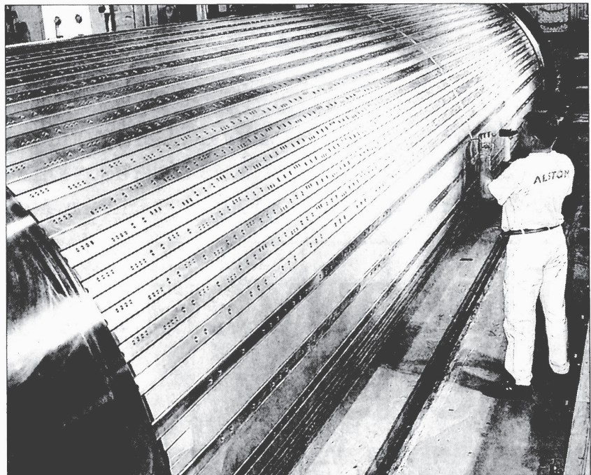
■ La fabrication d'un rotor chez Alstom Power à Belfort.
